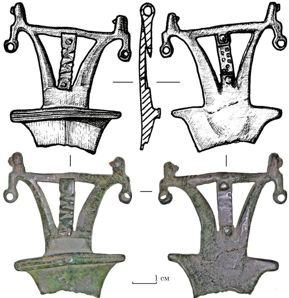
Рис. 1. Уламок Т-подібної фібули із поселення Шедієве, уроч. Ігнатівка
