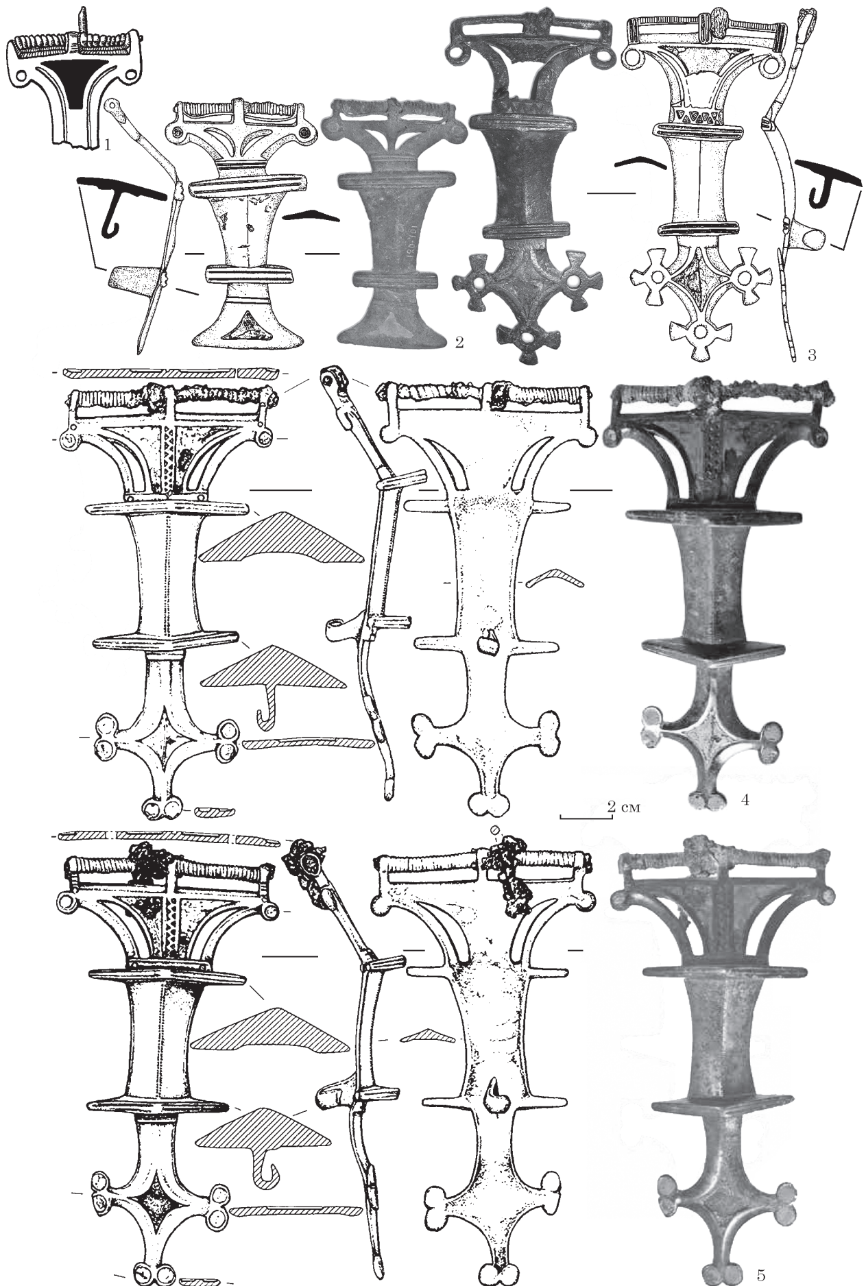
Рис. 3. Коло найближчих прототипів Т-подібній фібулі із поселення Шедієве, уроч. Ігнатівка. 1 — Григорівка; 2 — Дуна; 3 — Камунта; 4, 5 — Брянський скарб; 6 — Верхне Погромне; 7 — Паніковець 1
