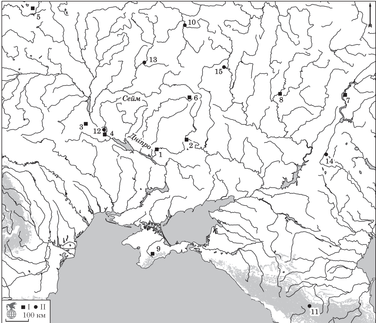
Рис. 4. Карта поширення найближчих аналогів та прототипів Т-подібної фібули із поселення Шедієве, уроч. Ігнатівка. Умовні позначення: I — аналоги; II — прототипи. Пам'ятки: 1 — Шедієве, уроч. Ігнатівка; 2 — Нижній Бишкін; 3 — «Васильківський» район; 4 — «Канівський» район; 5 — Сватки; 6 — Нагольне; 7 — Подгорное II; 8 — Малик; 9 — Нейзаг; 10 — Дуна; 11 — Камунга; 12 — Григорівка; 13 — Брянський скарб; 14 — Верхне Погромне; 15 — Паніковець 1
