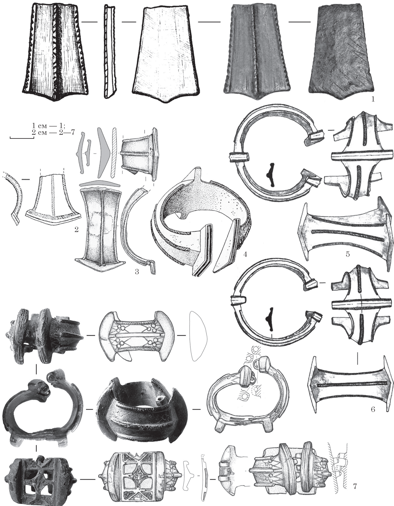
Рис. 5. Знахідка із Шедієвого та певні аналогії серед гребінчастих браслетів кола східноєвропейських варварських виїмчастих емалей: 1 — Шедієве, уроч. Ігнатівка; 2 — Заозер'я; 3 — Курська область; 4 — Пакачіне-Дембай; 5, 6 — Журавка / Лук'янчиков; 7 — Паніковець 1
