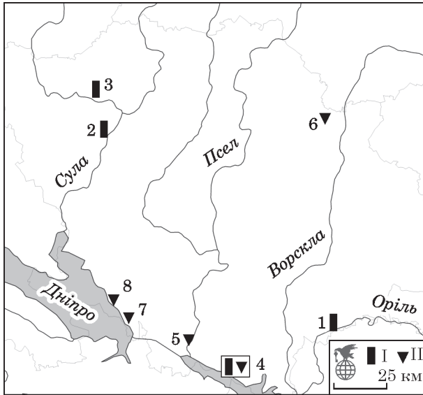
Рис. 6. Карта поширення прикрас та посуду київської традиції на пам'ятках черняхівської культури в Полтавській області. Умовні позначення: I — знахідки кола східноєвропейських варварських виїмчастих емалей заключного етапу; II — черняхівські пам'ятки із знахідками кераміки київської культури. Пам'ятки: 1 — Шедієве, уроч. Ігнатівка; 2 — Плютенці; 3 — Сухоносівка / Постав-Муки; 4 — Компанійці; 5 — Дмитрівка III; 6 — Перещецино 2; 7 — Максимівка; 8 — Радущівка
