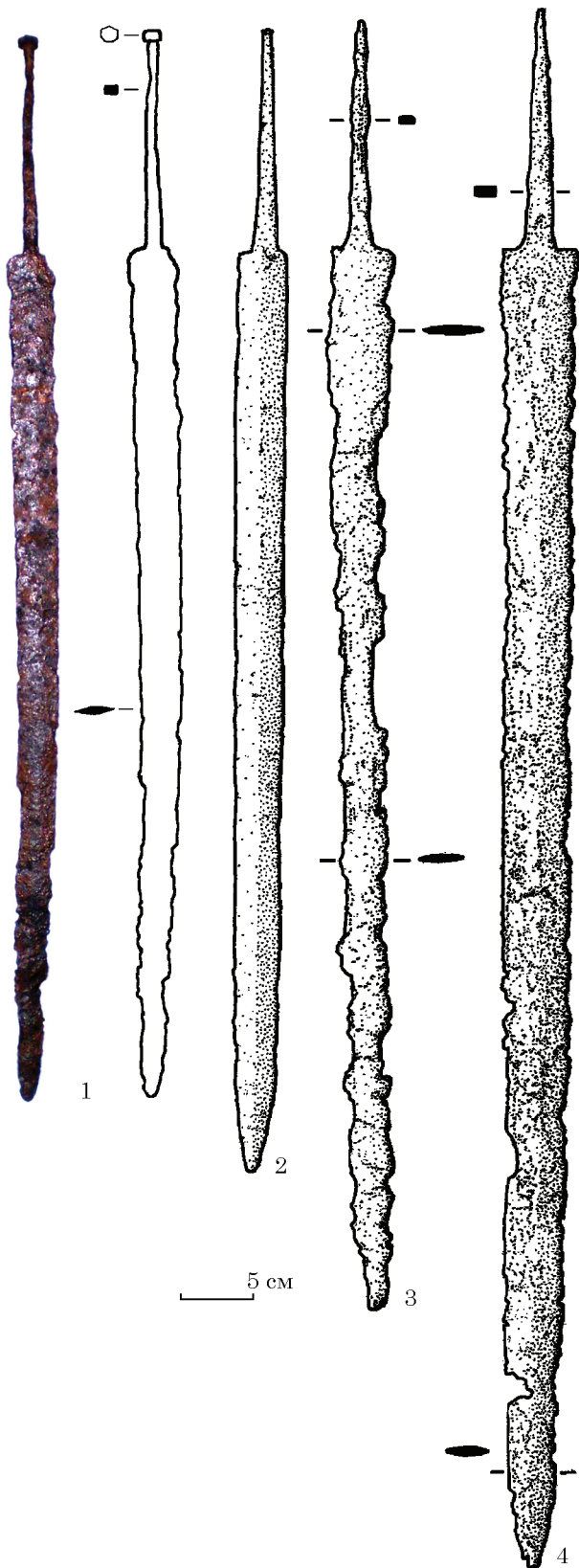
Рис. 7. Меч з Червоного Маяка і spatha: 1 — Пропасна балка, випадкова знахідка; 2 — Ньюстед; 3 — Камелон; 4 — Роттвайл (2—4 — за: Bishop, Coulston 1993)
