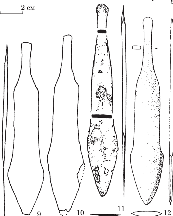
Рис. 53. Ножі типу IX.5: 1 — Фрунзе 8/4; 2 — Говору- ха 1/3; 3 — Олександрівськ 10/13; 4 — Блаківка 1/9; 5 — Новомикільське 1/10; 6 — Новомикільське 1/3; 7 — Сватове 10/1; 8 — Христофорівка 6/16; 9 — Степовий 3/5; 10 — Жолобок 3/6; 1977; 11 — Кривий Ріг, Рибасове II 4/10; 12 — Окниця 3/15 (1 — Братченко 1976; 2, 4 — Смирнов 1996; 3 — Післарій 2008; 5, 6 — Братченко, Швецов 1991; 7 — Братченко 2004; 8 — Шапошникова и др. 1973; 9 — Санжаров 2010; 10 — Післарій и др. 1977; 11 — Мельник, Стеблина 2012; 12 — Ключко Е. 1990)
