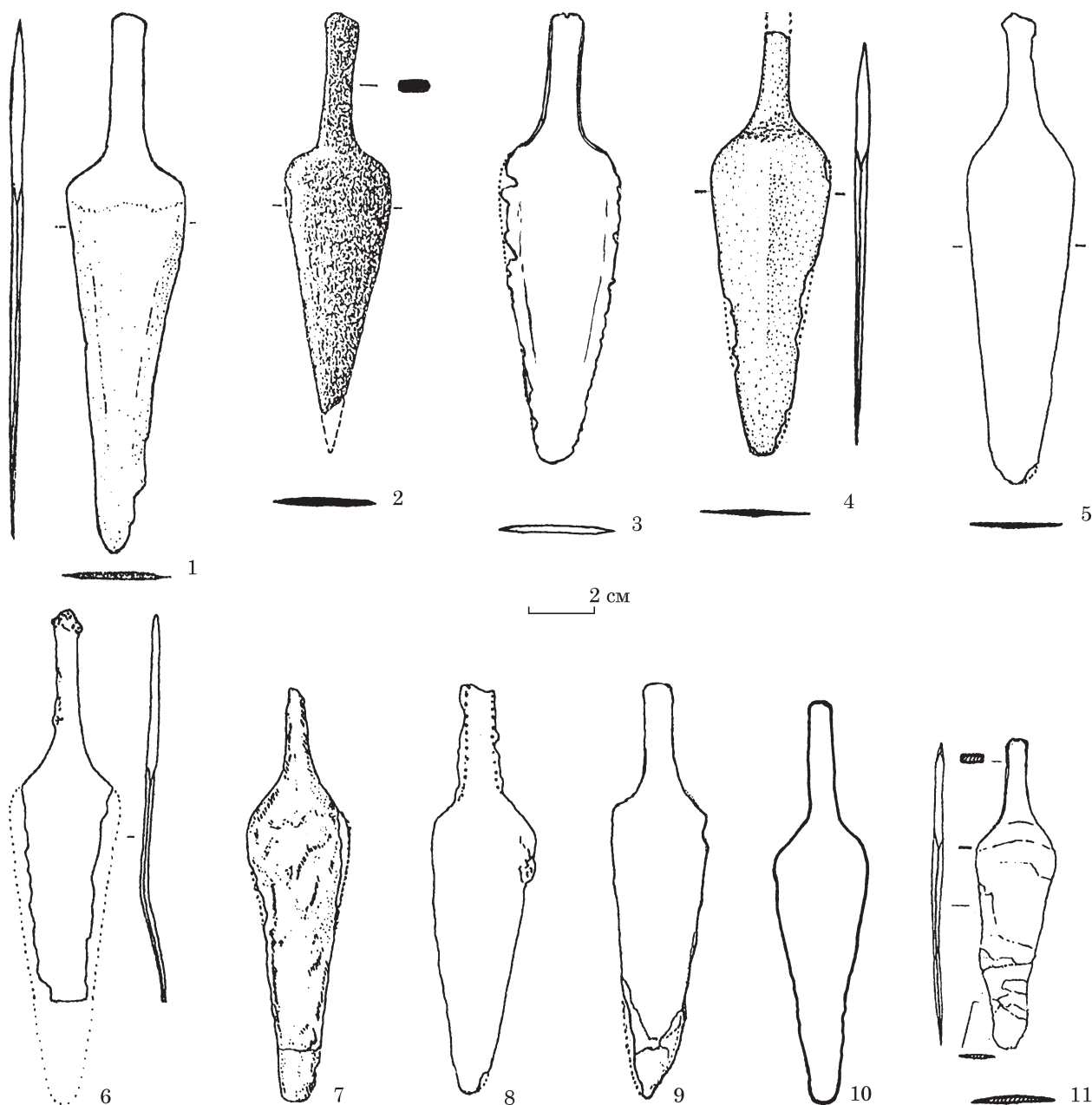
Рис. 18. Ножі типу VI.2: 1 — Луганськ (ВСП) 1/1; 2 — Кривий Ріг (Войкове) 2/23; 3 — Павлиш 1/1; 4 — Широке 3/14; 5 — Царівка 4/6; 6 — Василівка 8/9; 7 — Болотне 14/28; 8 — Сергіївка II 3/3; 9 — Бабенкове 1/19; 10 — Бешчасна Могила; 11 — Садове 2/1 (1 — Гладких и др. 1974; 2, 4 — Мельник, Стеблина 2012; 3 — Бокий 1969; 5 — Братченко и др. 1980; 6 — Kaiser, Plešivenko 2000; 7 — Генинг, Корпусова 1989b; 8 — Кубышев и др. 1984; 9 — Щепинский, Черепанова 1969; 10 — Самоквасов 1905; 11 — Евдокимов и др. 1992)
