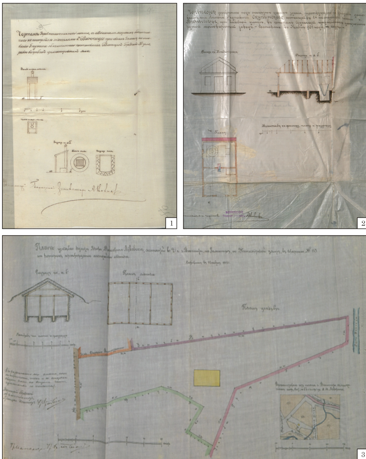
Рис. 16. Господарчі споруди присадибних ділянок: 1 — план-проект уніфікованого відхожого місця; 2 — план-проект миловарні; 3 — план-проект льодовні (за: 1 — Протоколи... 1881—1896; 2 — Пляны... 1901; 3 — Прошения... 1901—1914)
