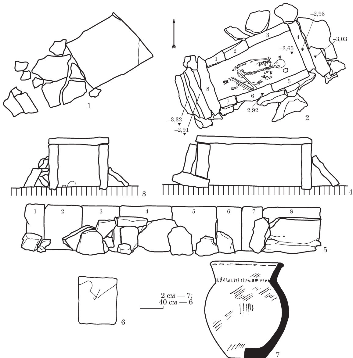
Рис. 7. Село Львове, кург. 8, пох. 3: 1 — перекриття скрині; 2 — план поховання у скрині; 3—5 — розрізи та розгортка скрині; 6 — прокреслений орнамент на західній плиті; 7 — горщик з поховання (за: Тереножкин и др. 1973; рисунок горщика Ю. Я. Рассамакіна)
