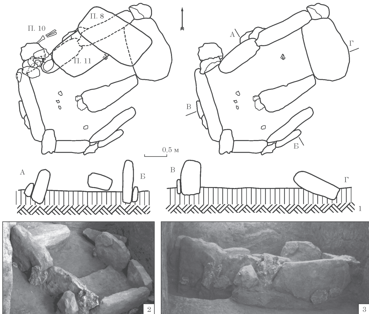
Рис. 5. Село Новопилипівка, гр. «Аккормень І» кург. 11, пох. 14 (за: Вязьмитина 1952)
