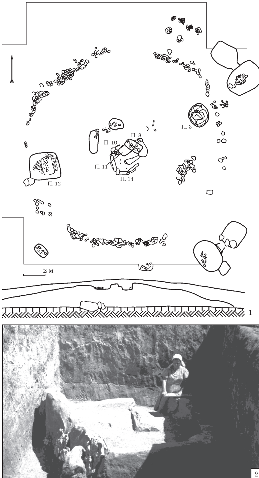
Рис. 4. Село Новопилипівка, гр. «Аккермень І» кург. 11: 1 — загальний план і профіль кургана; 2 — фото пох. 14 (за: Вязьмитина 1952)
