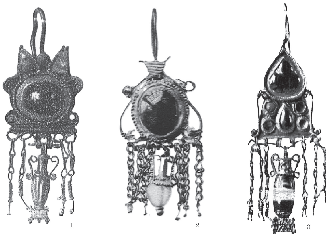
Рис. 5. Композитні сережки: 1 — поховання 47 (5) некрополя Пантікапея на Глиниці; 2 — Ольвія, поховання, розкопане селянами в 1891 р.; 3 — могила 44 некрополя Пантікапея на горі Мітрідат (за: 1 — Шкорпил 1913; 2 — Орешников 1894; 3 — Шкорпил 1905)
